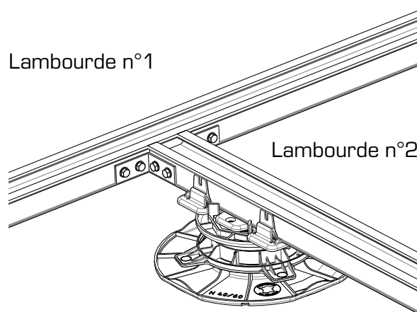
Assemblage avec équerre horizontale
